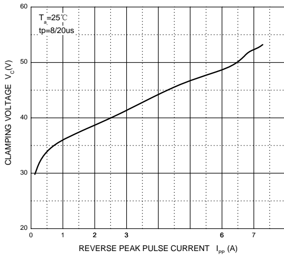
V_C — I_{PP}
