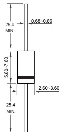
DO-15 Unit:mm
